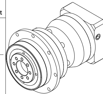
OPH雙級尺寸圖
